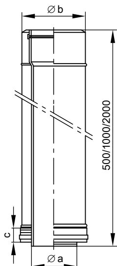
Труба для наружной стены
