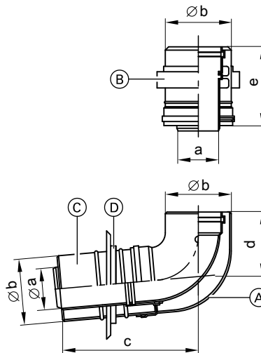
Модульный размер Ø 100 мм
