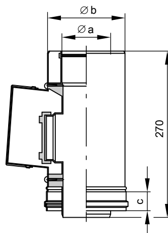
Ревизионный элемент наружной стены
