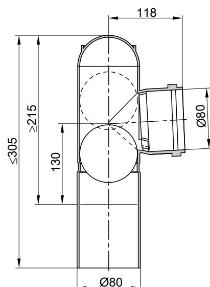
Модульный размер Ø 80 мм
