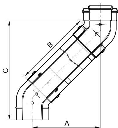
Модульный размер Ø 60 мм
