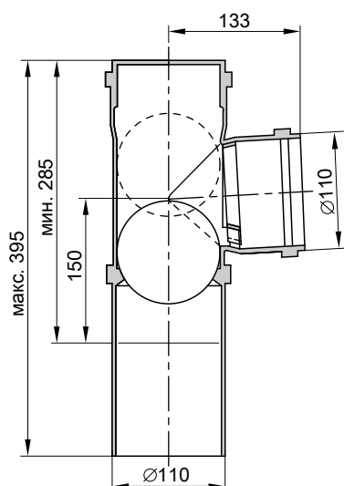
Модульный размер Ø 100 мм
