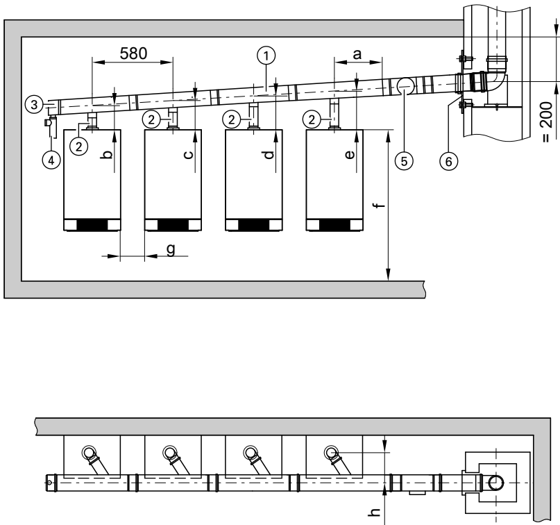
Vitodens 200-W
