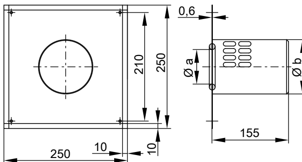
Стенная диафрагма LAS в системе связанных помещений
