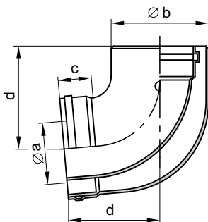
Колено наружной стены 87°
