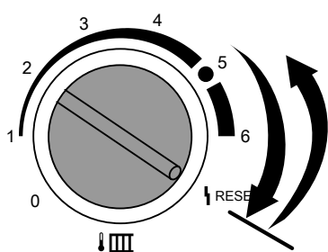
Ⓐ Ограничитель температуры
