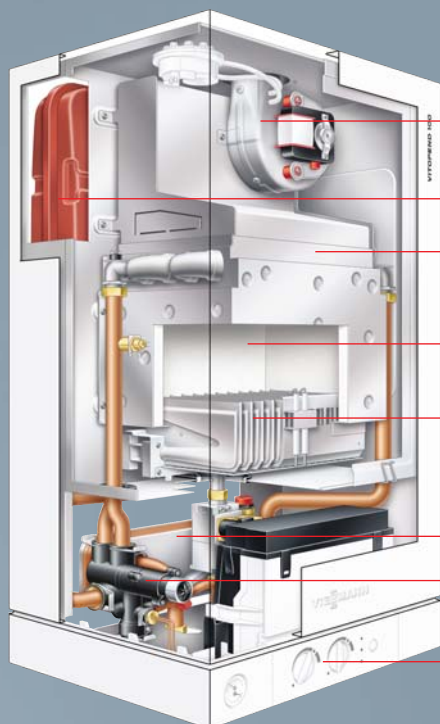
Комбинированный котел с закрытой камерой сгорания
