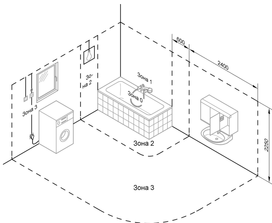
Зоны электрозащиты
