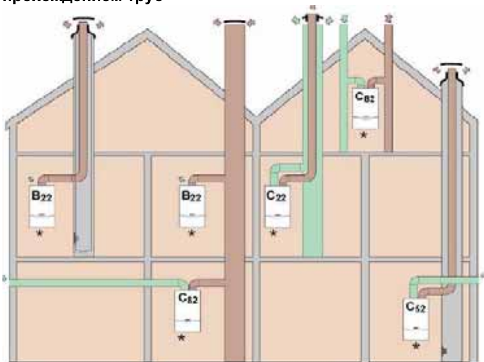
Системы с раздельным прохождением труб
