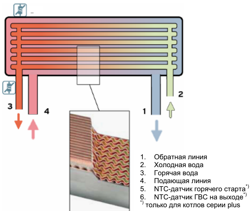
Вторичный теплообменник с NTC-датчиком (котлы серии plus)
