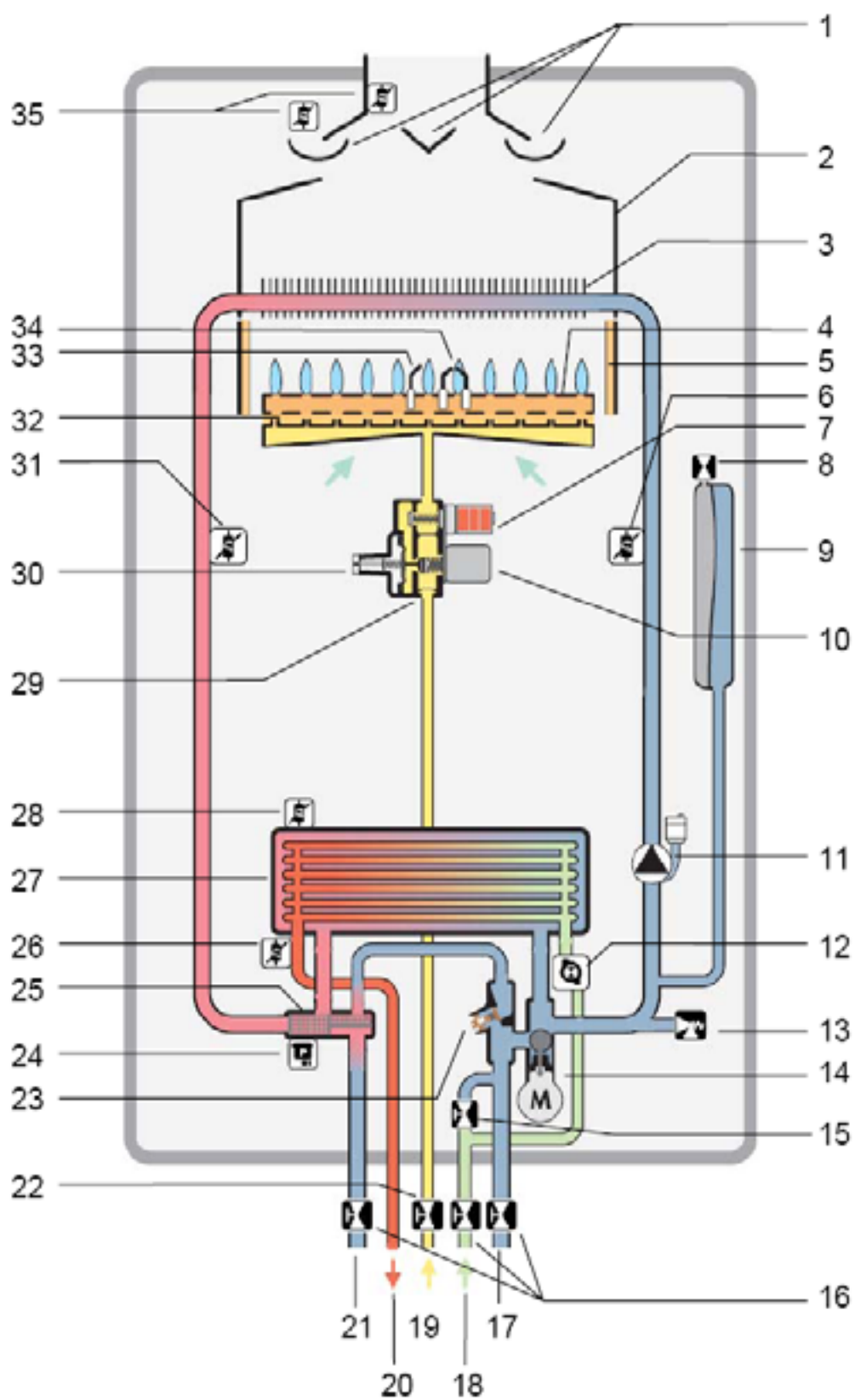
Функциональная схема atmoTEC plus VUW INT ...
