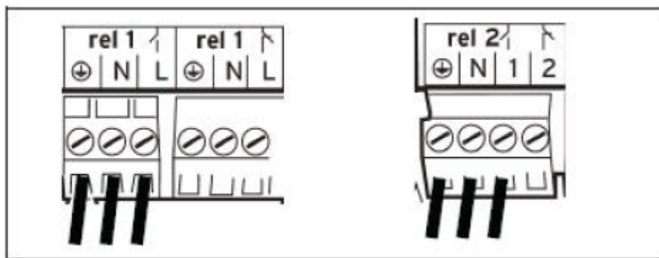
Подключение внешнего электромагнитного клапана
