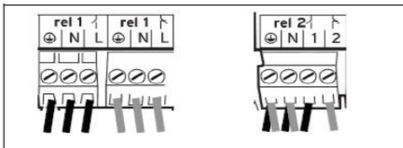
Подключение вытяжного колпака / клапана отходящих газов
