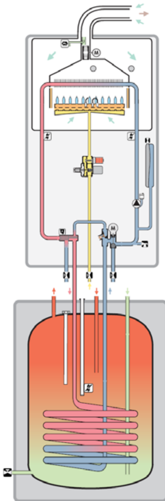
Функциональная схема turboTEC plus VU INT ... с водонагревателем VIH R 120
