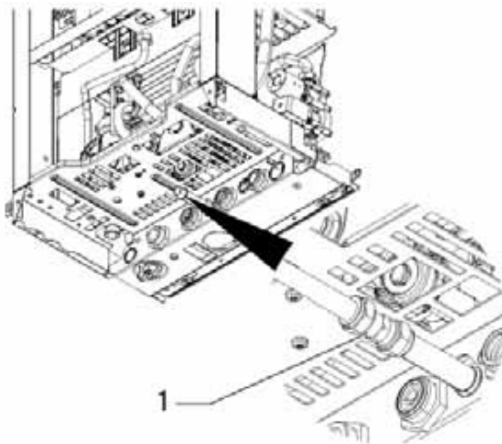
Патрубок подключения газа
