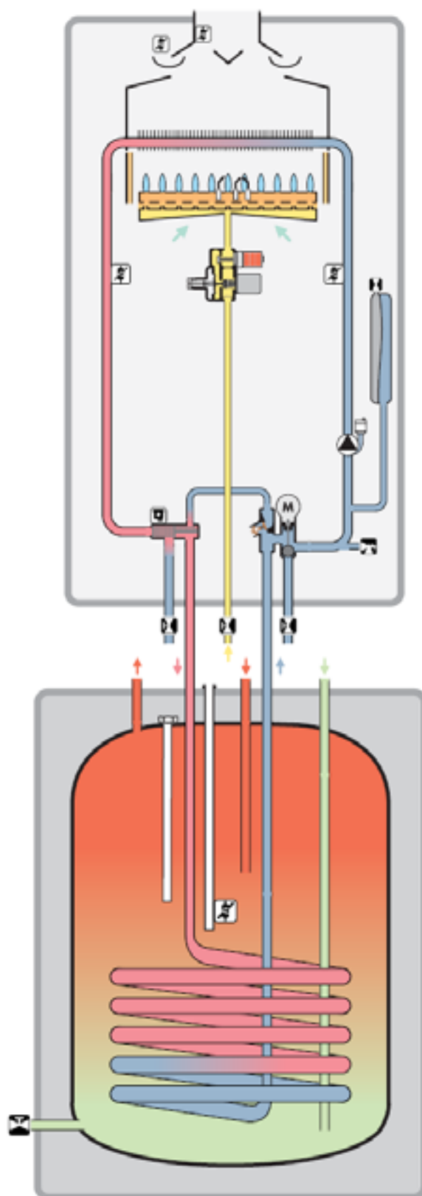
Функциональная схема atmoTEC plus VU INT ... с водонагревателем VIH R 120
