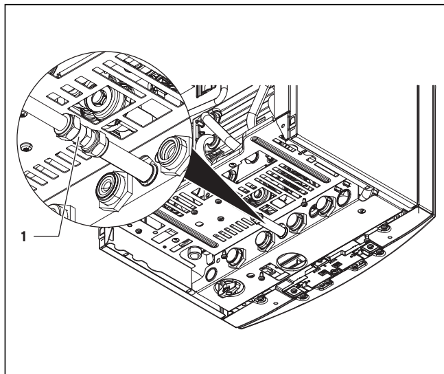
Рис. 5.1 Подсоединение газа
