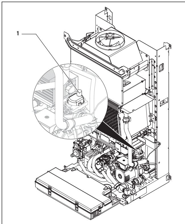
Рис. 6.1 Быстродействующий воздухоотводчик
