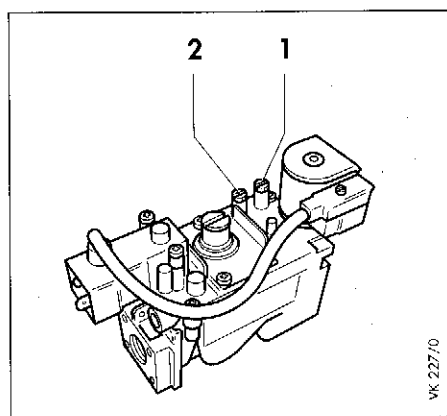
Рис. 8.6 Штуцеры для измерения давления на входе у котлов VK 30E - 45E
