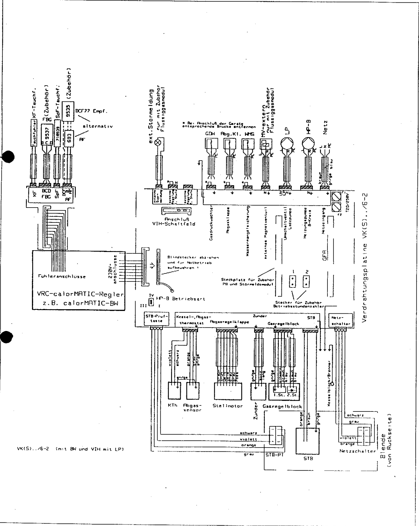
Abb. 11.1 Verdrahtungsplan
