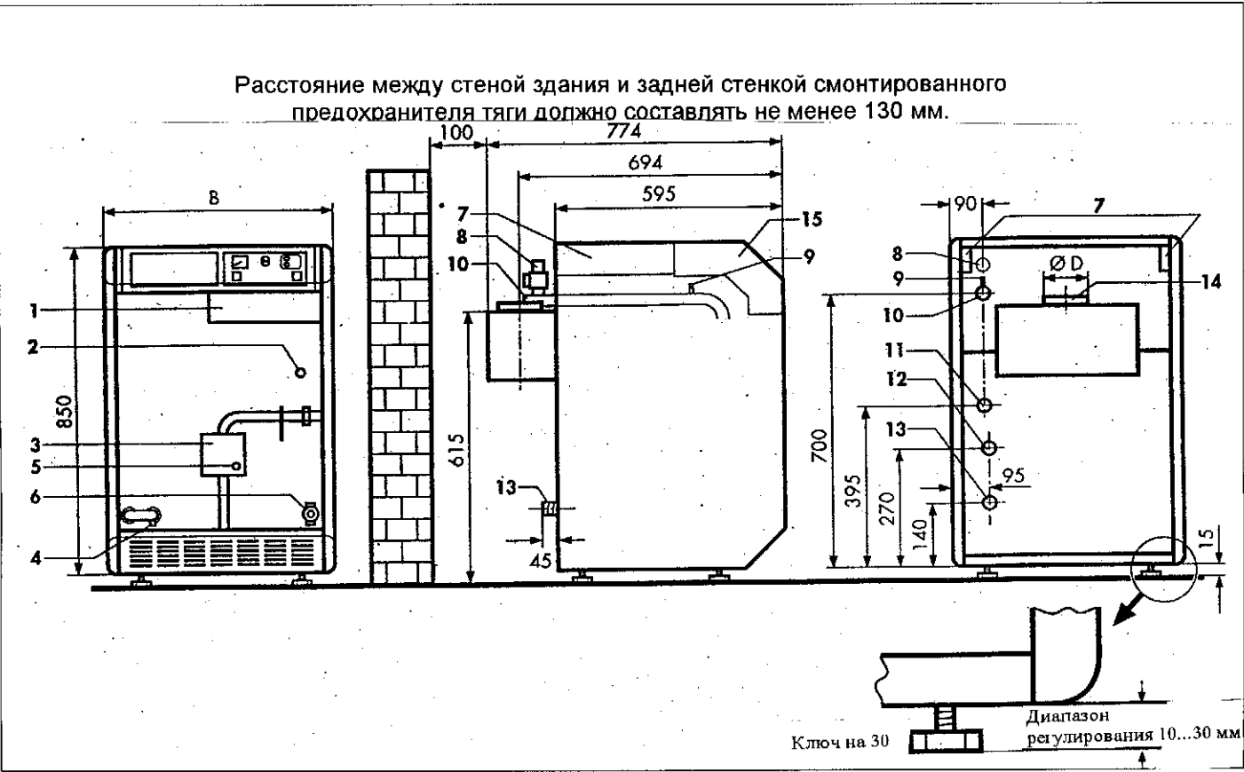
Рис.4.1 Размеры
