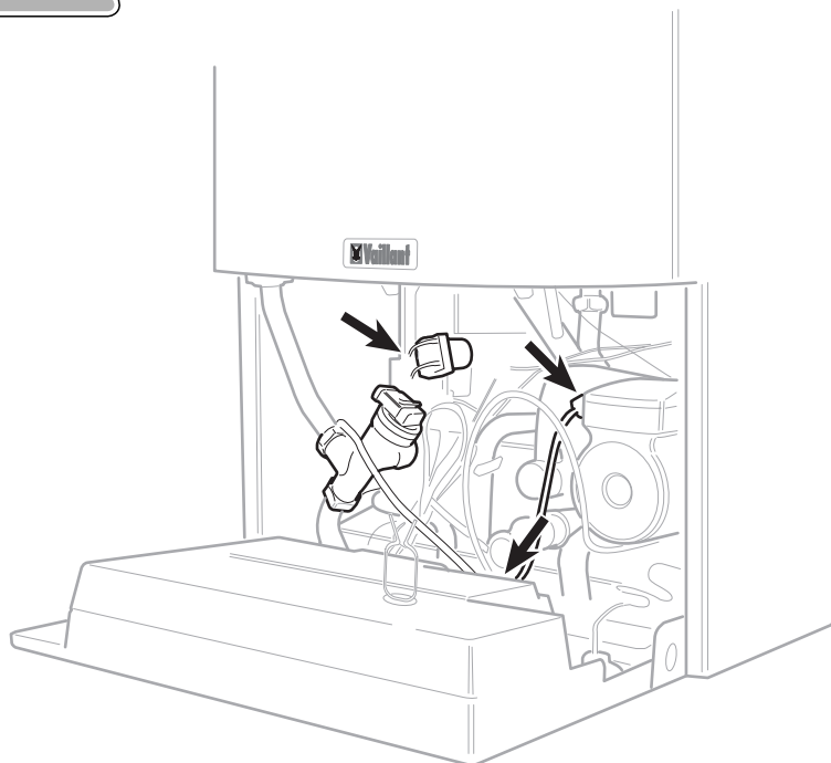
Рис. S.1: Опасность поражения электрическим током
