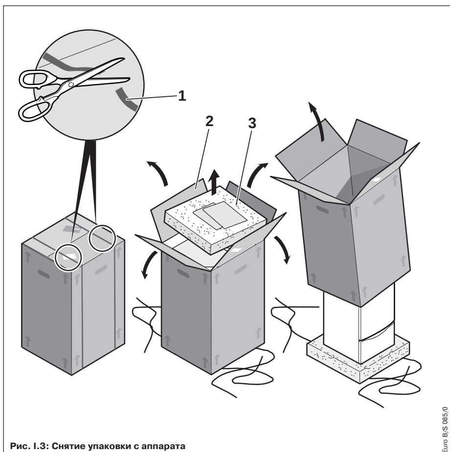
Рис. 1.3: Снятие упаковки с аппарата
