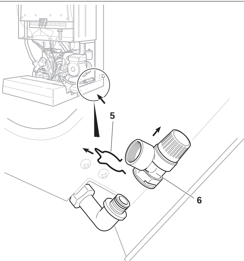
Рис. Е. 17: Предохранительный клапан
