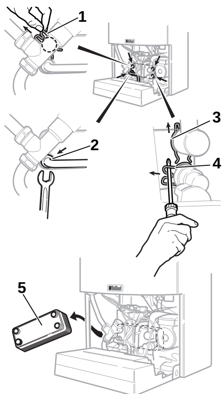
Рис. Е. 16: Вторичный теплообменник
