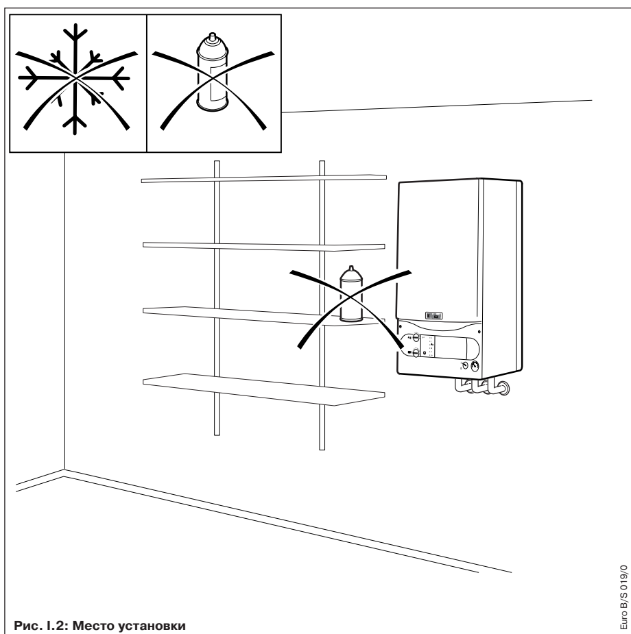
Рис. 1.2: Место установки
