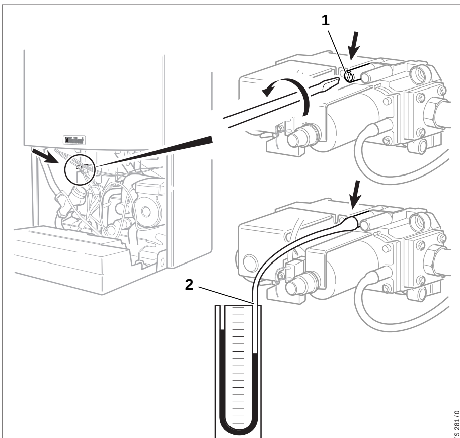
Рис. Г. 1: Проверка давления газа (давления истечения) в подводящем газопроводе
