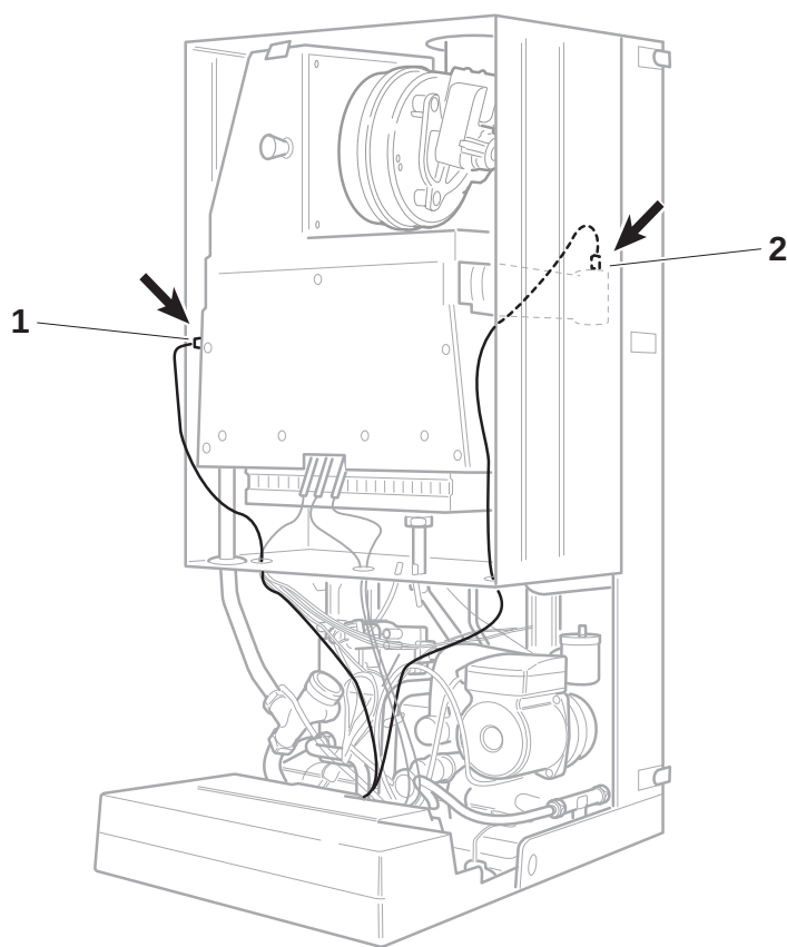
Рис. Е.6: Датчики NTC
