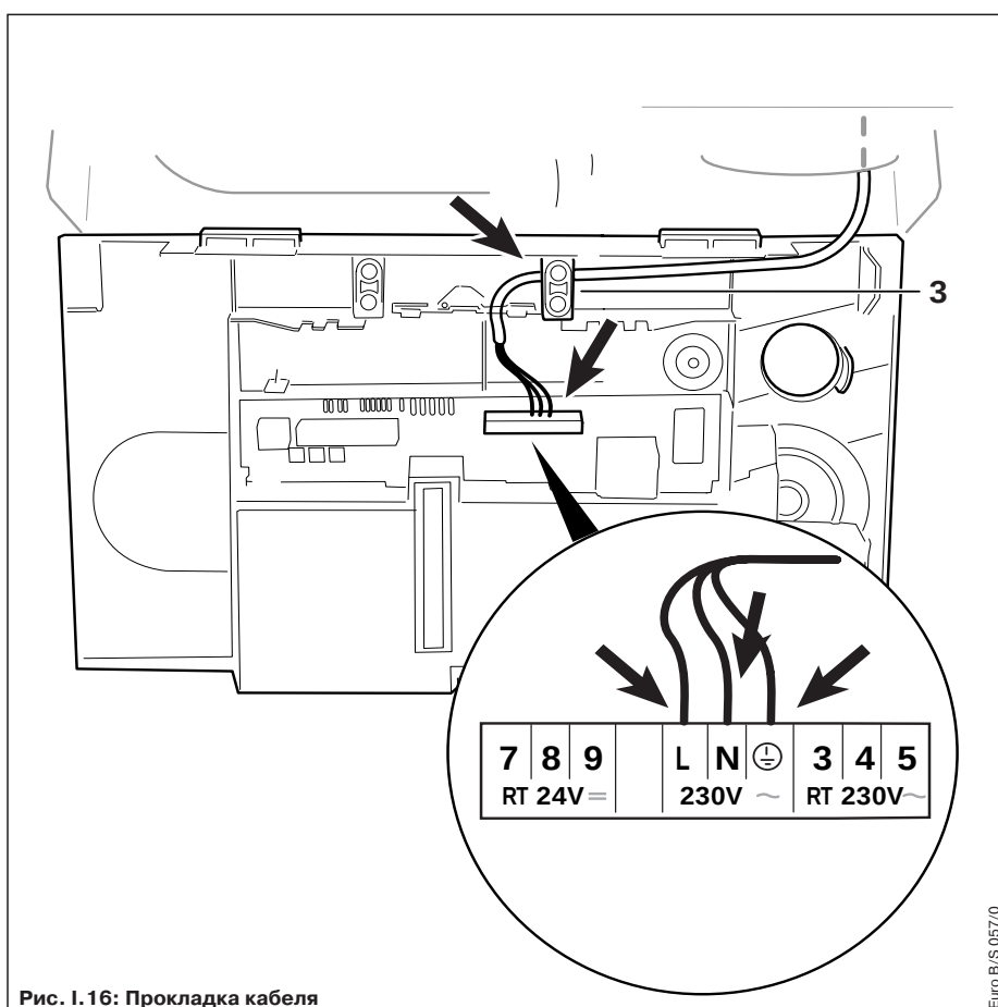
Рис. I. 16: Прокладка кабеля
