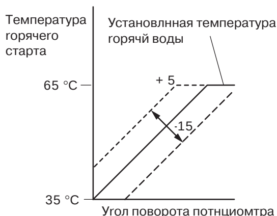
Рис. We.4: Регулировка температуры горячего пуска
