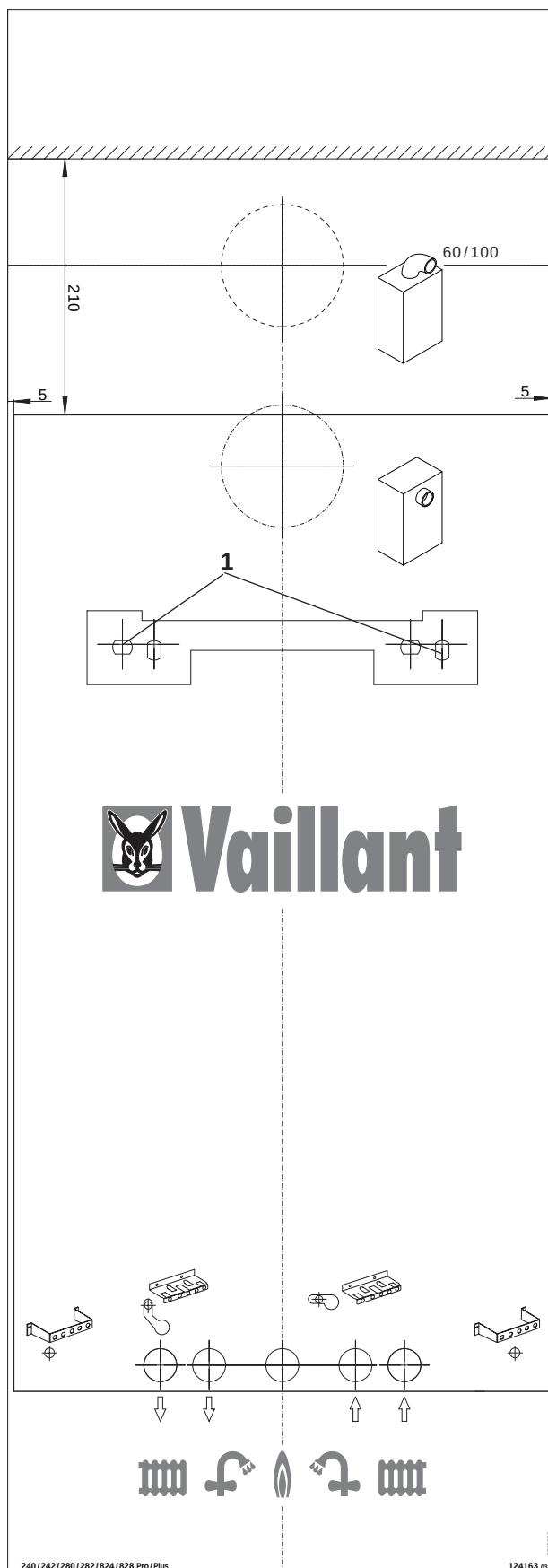
Рис. 1.6: Монтажный шаблон
