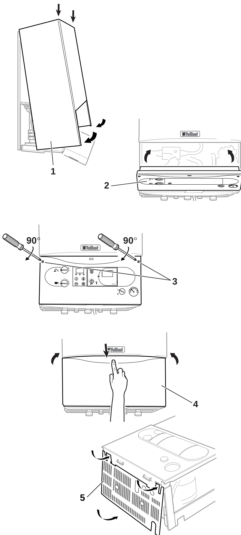
Рис. I.23: Установка облицовки аппарата на место
