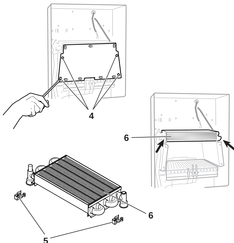
Рис. Е.7: Первичный теплообменник
