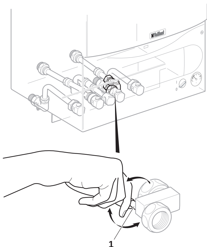
Рис. We.3: Регулировка расхода горячей воды
