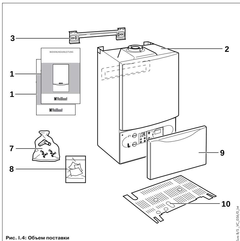
Рис. I.4: Объем поставки
