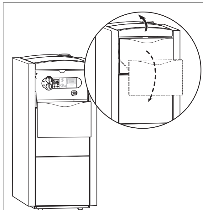
Рис. 3.1 Открывание дверцы облицовки
