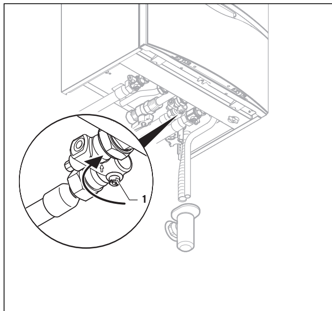
Рис. 2.3 Закрывание запорного вентиля холодной воды (не касается VU 466 и 656)
