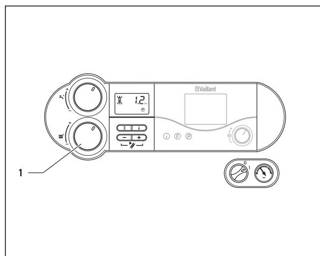
Мал. 4.12 Вимкнення режиму опалення (літній режим) (тут показаний: atmoTEC/turboTEC plus)
