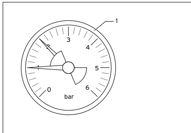
Fig. 4.4 Controllo della pressione di riempimento dell'impianto di riscaldamento (manometro sul posto)
