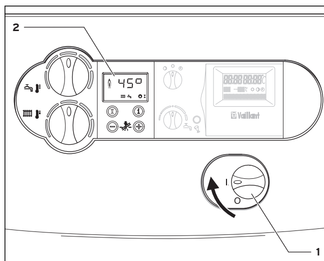
Fig. 4.5 Conectarea aparatului
