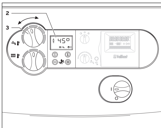
Attēls 4.6 Uzkrāšanas tvertnes temperatūras iestatīšana (tikai, ja ir pievienota karstā ūdens tvertne)
