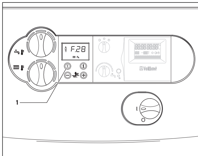
Рис. 4.13 Устранение неисправностей
