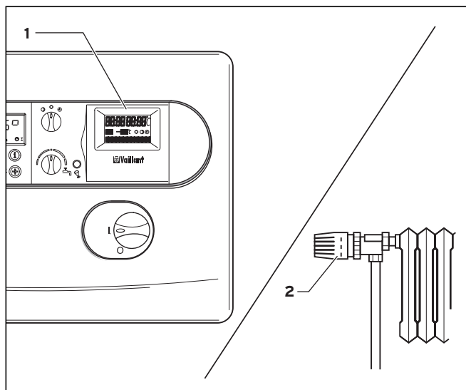
Рис. 4.10 Настройка регулятора температуры помещения/регулятора в зависимости от погодных условий
