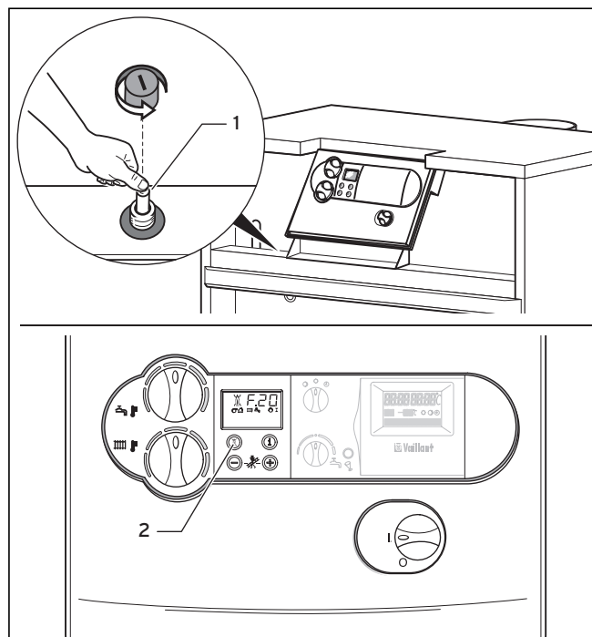
Рис. 4.12 Разблокировка после отключения по нехватке воды
