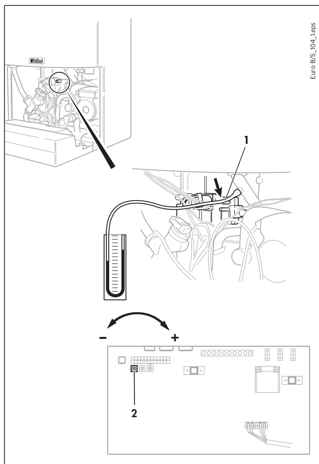
Рис. 4.5 Проверка и регулировка режима частичной мощности отопительной системы путем определения давления на соплах
