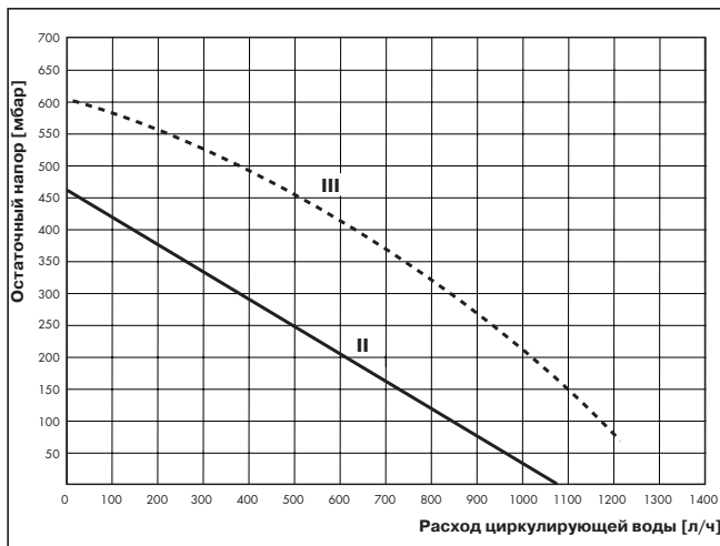
Рис. 6.4 Характеристика насоса
