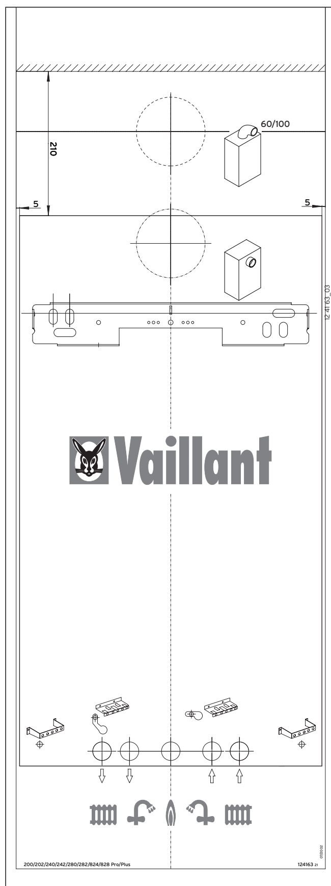
Рис. 3.2 Монтажный шаблон
