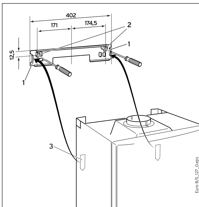
Рис. 3.7 Навеска аппарата
