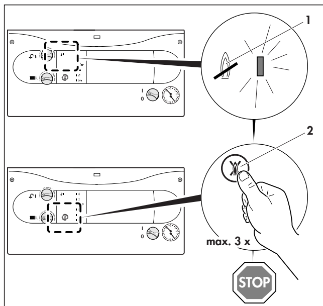
Fig. 10: Înlăturarea defecțiunilor
