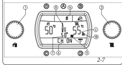
Működés téli modalitásban külső szondával (opcionális)
