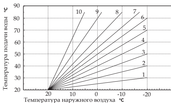
Кривые компенсации
