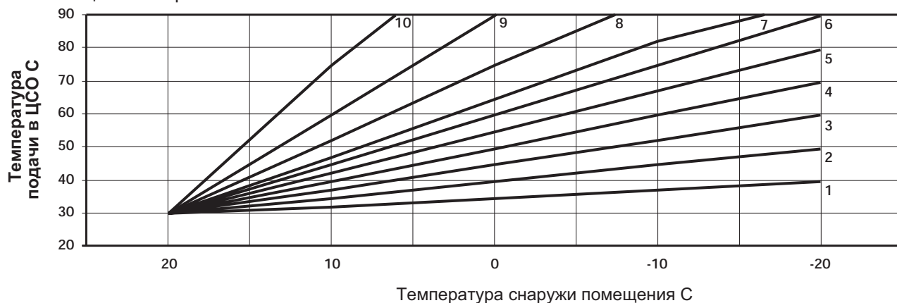
Компенсационные кривые
