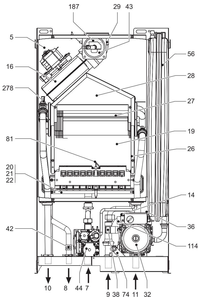
рис. 26 - Общий вид
