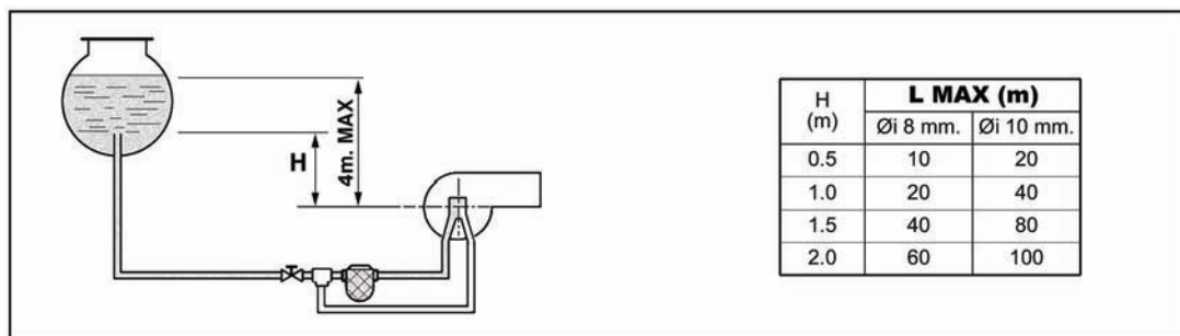
рис. 18 - Подача самотеком
