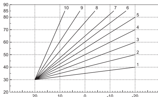
рис. 13 - Компенсационные характеристики
