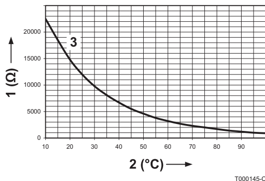
Рабочие диаграммы : Датчик температуры/Сопротивление, Ом
