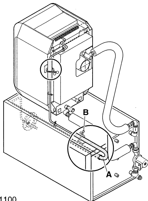
Датчик резервуара-аккумулятора
