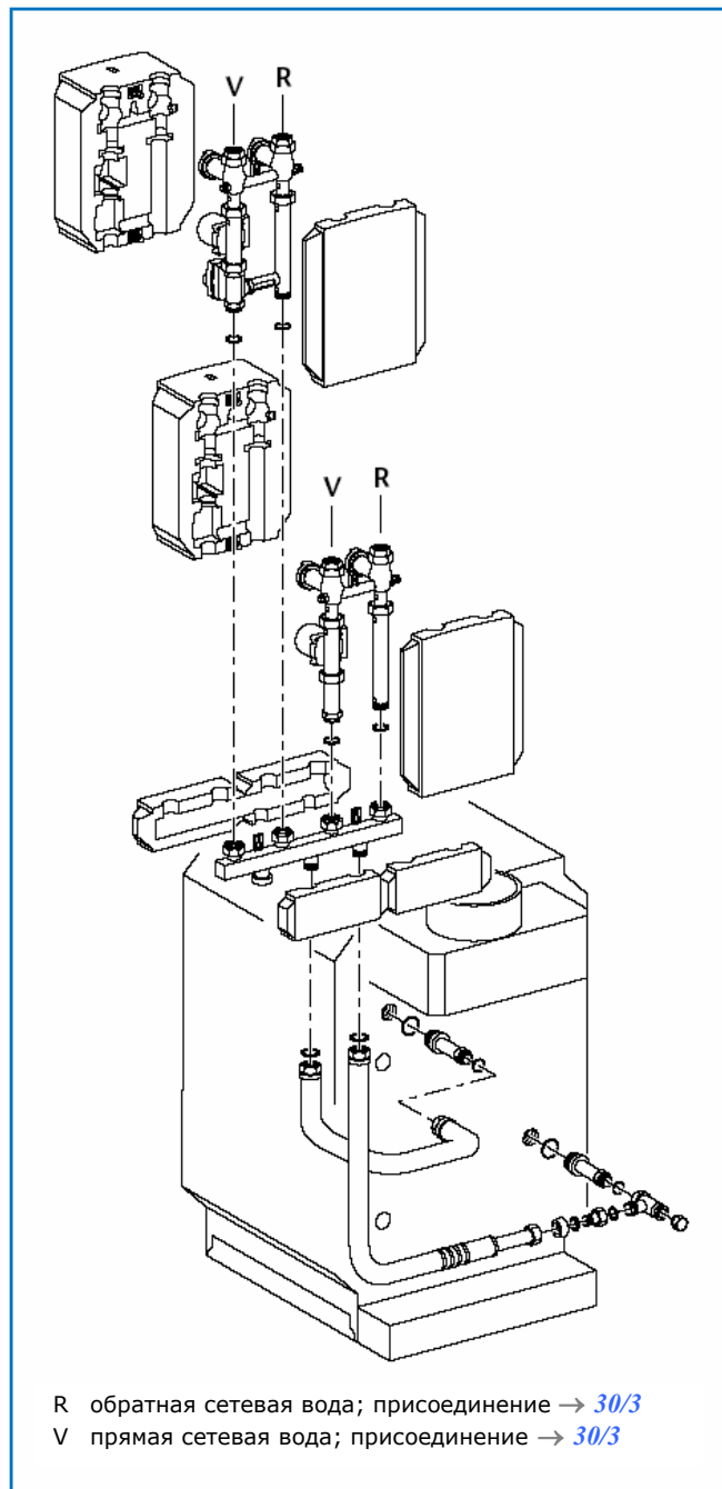
30/1 Газовый чугунный отопительный котел Logano G234 с системой быстрого монтажа RK 2M(-E)/G234
