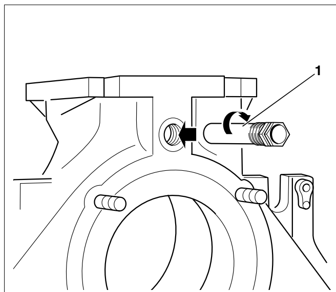
Рис. 25 Монтаж гильзы для датчиков
