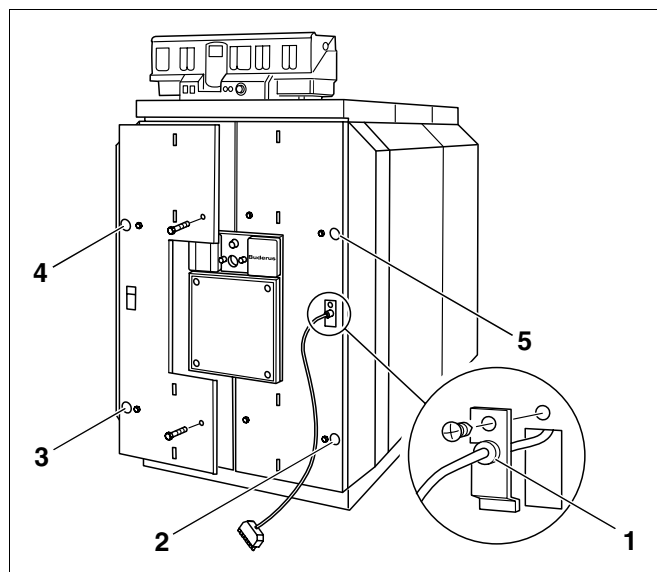
Рис. 57 Установка обшивки дверцы горелки
