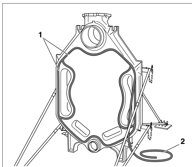
Рис. 16 Укладка уплотнительного шнура (шнур КМ)
