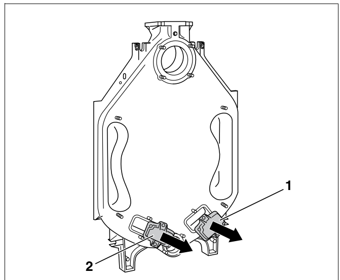
Рис. 10 Демонтаж крышек люков для чистки
