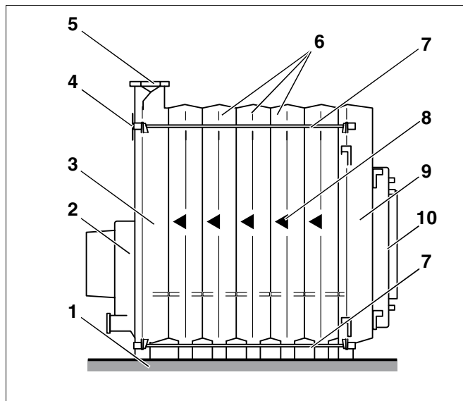
Рис. 8 Блок котла
