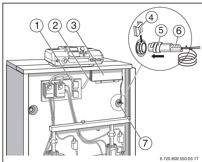
Рис. 23 Установка датчиков температуры
