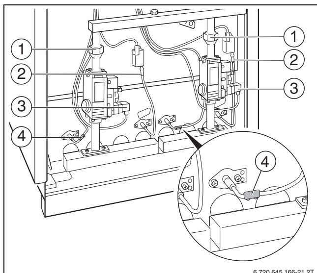
Рис. 57 Демонтаж горелки
