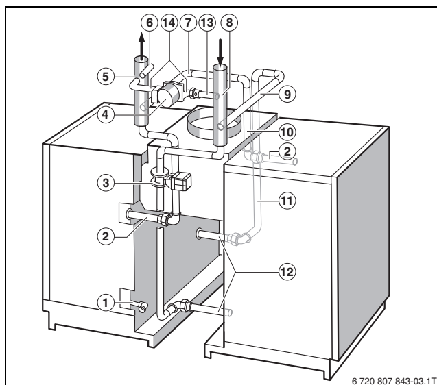
Рис. 14 Комплект подключения котла
