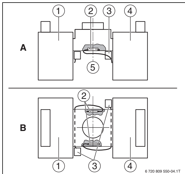
Рис. 33 Датчики температуры дымовых газов на сдвоенном котле
