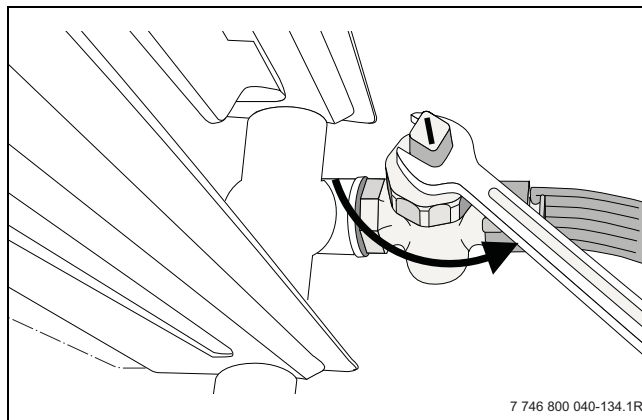
Рис. 51 Слив воды из отопительной системы при опасности заморозания
