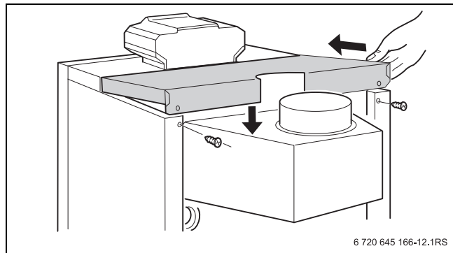
Рис. 29 Установка задней крышки котла
