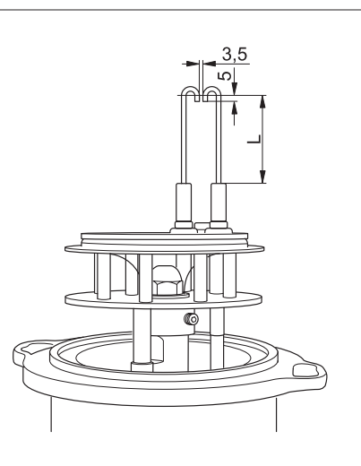
Рис. 5 Запальный электрод тип 3 – размер "L" (размеры в мм)
