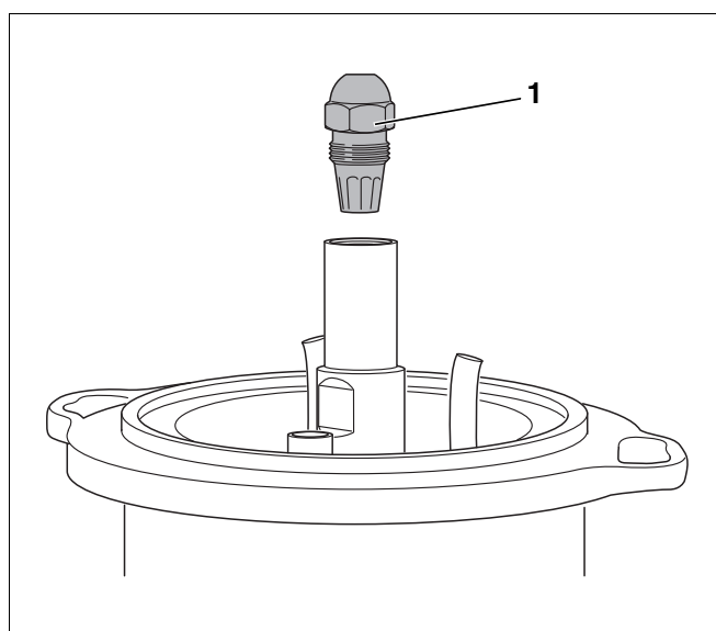
Рис. 29 Демонтаж форсунки
