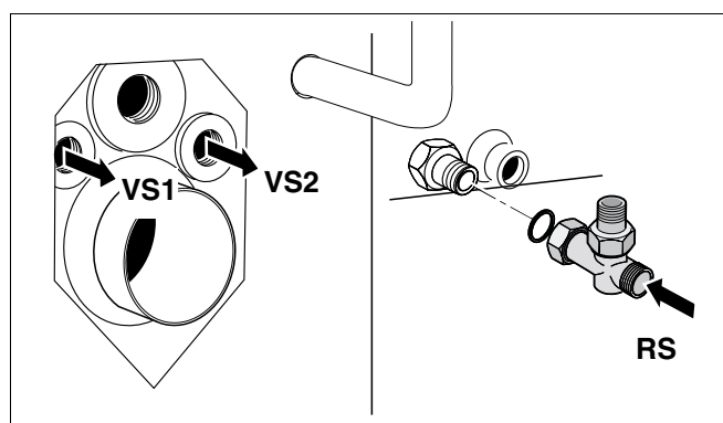
Рис. 20 Подключение бака-водонагревателя
