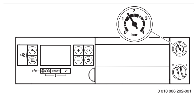
Рис. 4 Манометр для контроля рабочего давления при открытой крышке панели управления
