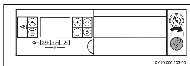
Рис. 8 Включение котла
