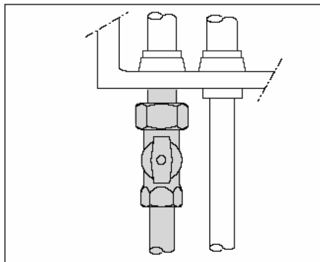
Рис. 5 Газовое присоединение
