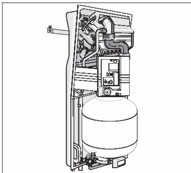
Рис. 3 Монтаж
