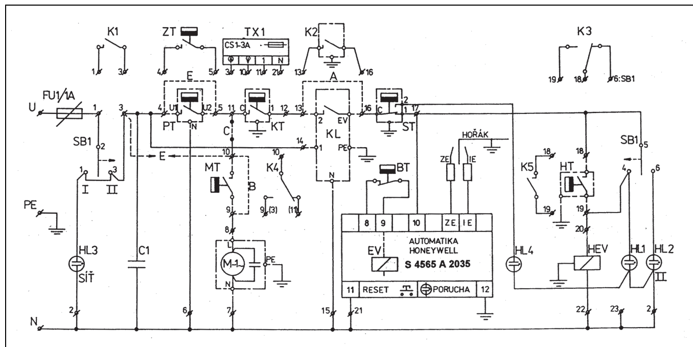
Рис. 11 Электрическая схема котлов FN 18-30 HN
