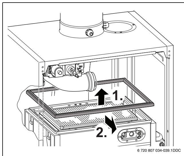
Рис. 55 Снятие уплотнения горелки
