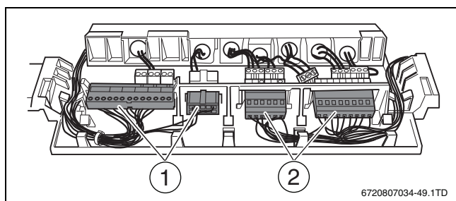
Рис. 27 Клеммные колодки
