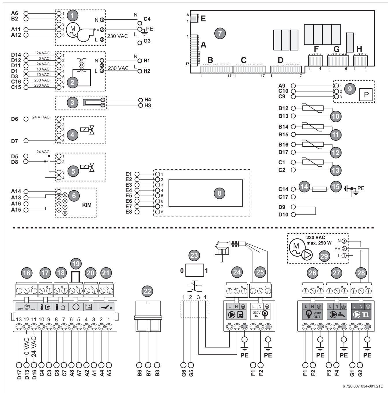
Рис. 5 Электрическая схема
