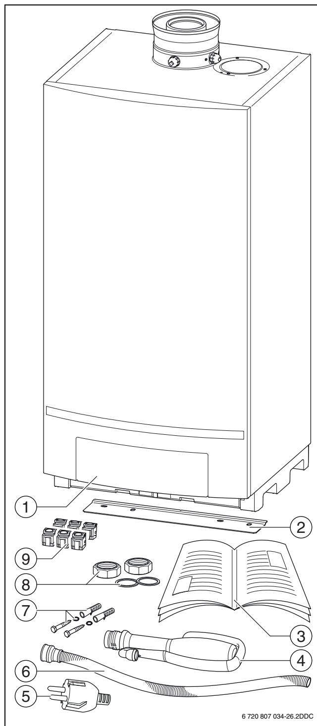
Рис. 1 Комплект поставки
