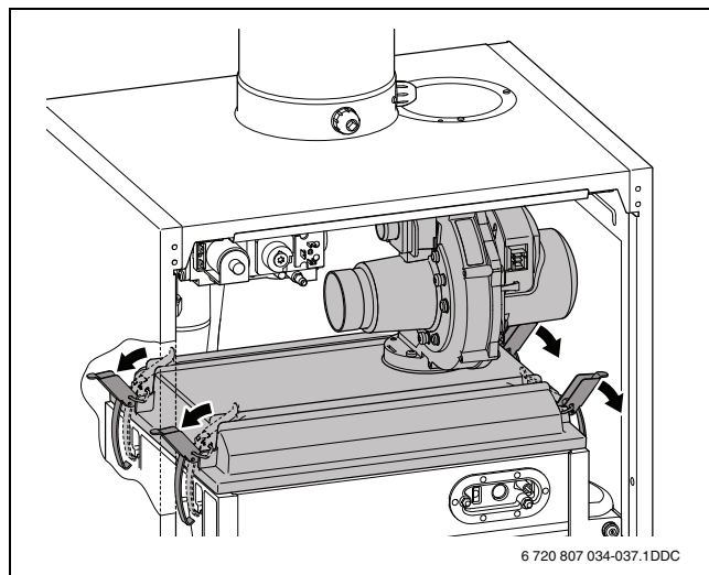
Рис. 53 Раскрытие защёлок
