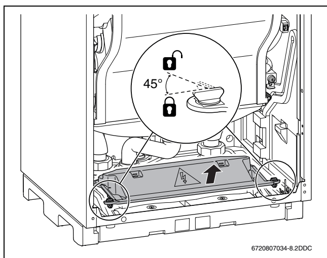
Рис. 26 Снятие крышки
