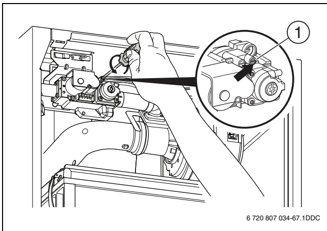
Рис. 65 Открытие штуцера измерения давления на форсунке (тип 70)
