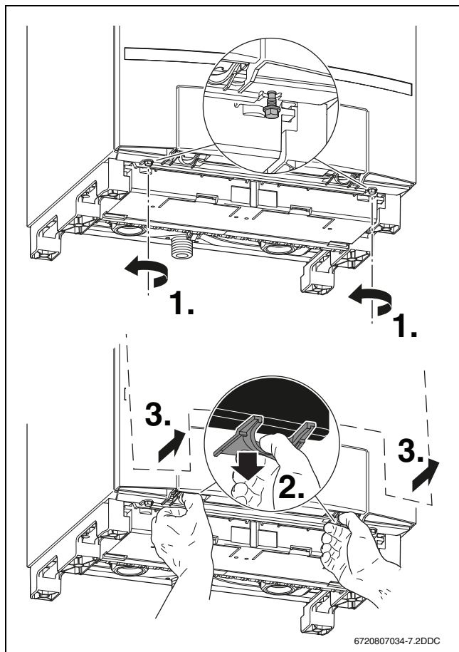
Рис. 2 Снятие облицовки
