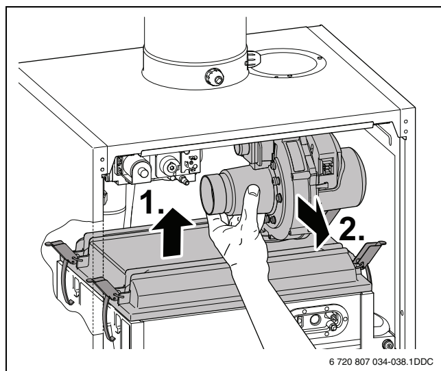
Рис. 54 Удаление газовоздушного блока с крышкой горелки
