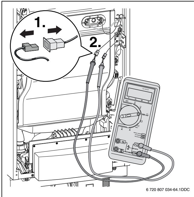
Рис. 48 Подключение мультиметра
