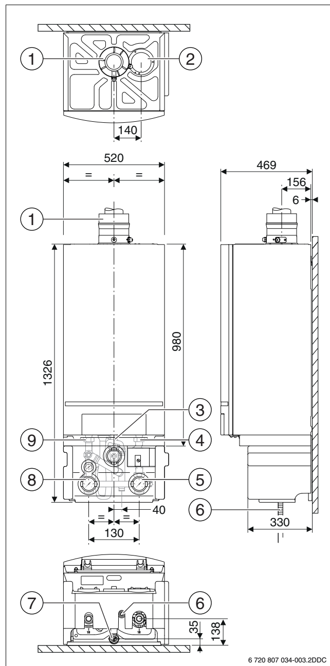
Рис. 3 Размеры [мм]
