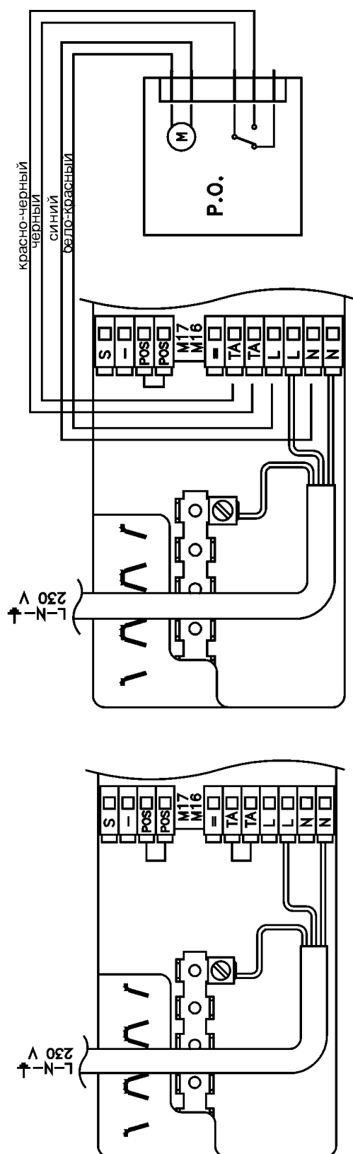
Базовое подключение
