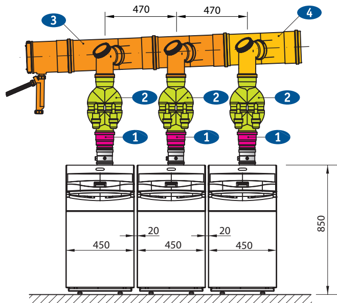
Подключение котлов POWER HT к единому вертикальному дымоходу
