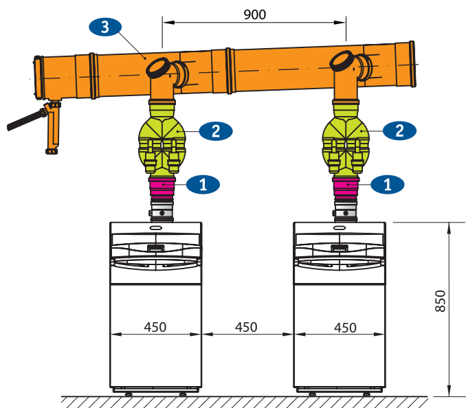
Подключение котлов POWER HT к единому вертикальному дымоходу
